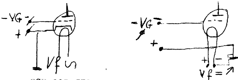
SCH 025 FIG 9:2 voorbeelden voor praktisch gebruik. De + aansluiting der -V_g dient altijd aan massa of aan katode te liggen, de - aan het rooster. Men kan de karakteristiek van een lamp meten door de -V_g te variëren en de anodestroomverandering te meten. Aangezien een
